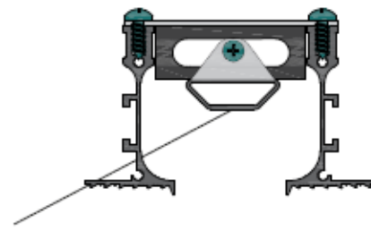
Дефлектор регулируемый
