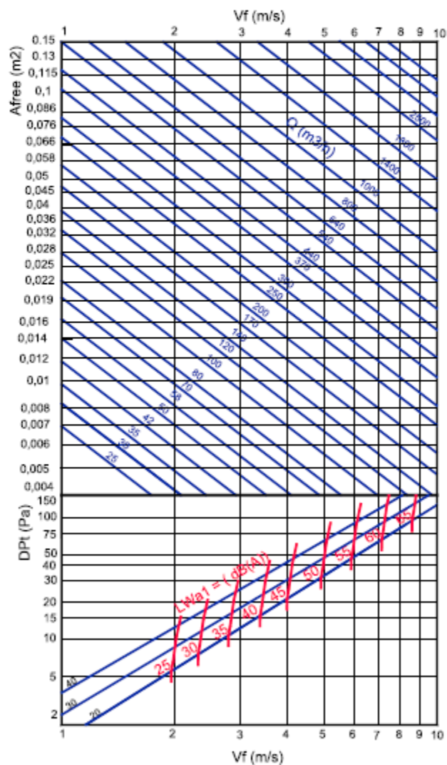
Расчетная скорость, потеря давления и уровень звуковой мощности
